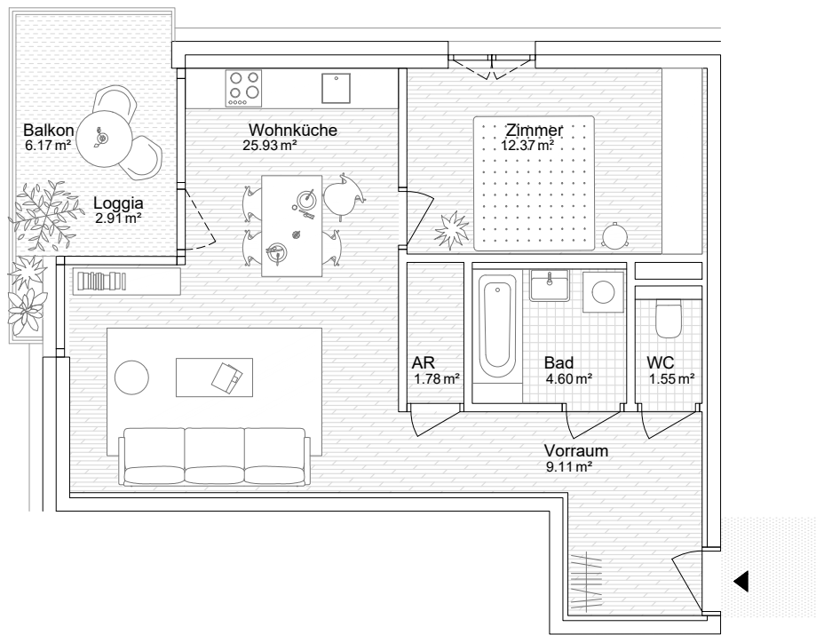
B Wohnung 55.35 m 2 +2.91 m 2 Loggia +6.17 m 2 Balkon
